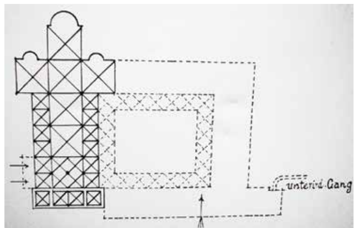
Ursprünglicher Grundriss der Kirche
